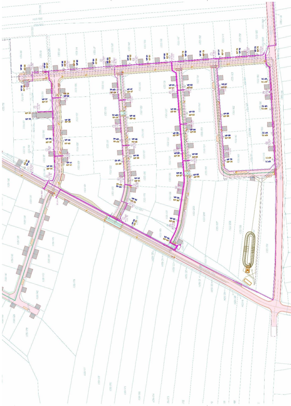
Příloha 1: Koordinační výkres
