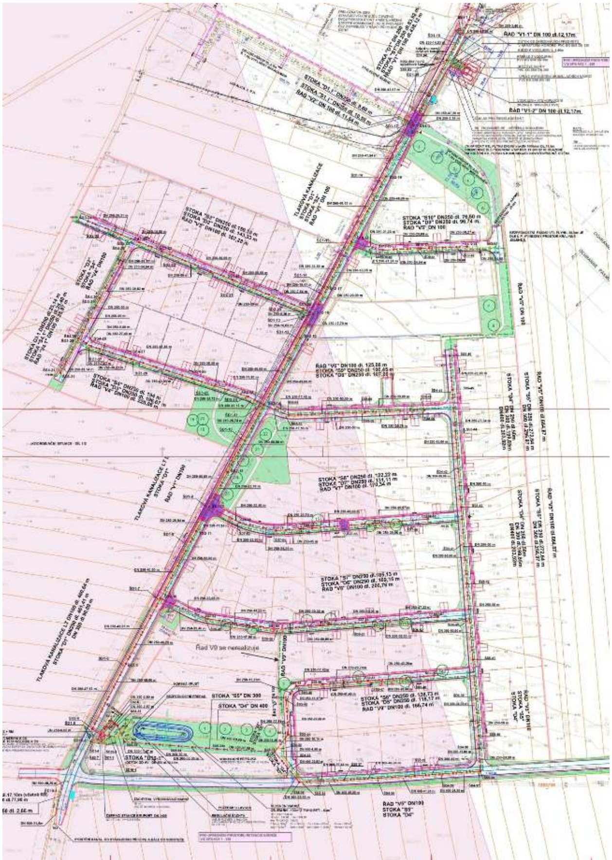
Príloha 1: Koordinační výkres
